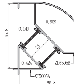
配套角码: GR5517
