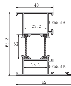
配套角码: JYL65M06
