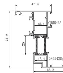
配套角码: JLL6536
