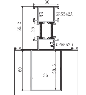
配套角码: GR5508 GR5518
